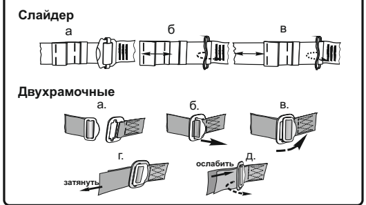
Рис. 6. Типы используемых пряжек, способы заправки пряжки
