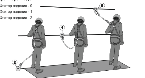
Рис. 4. Графическая схема к определению фактора падения
