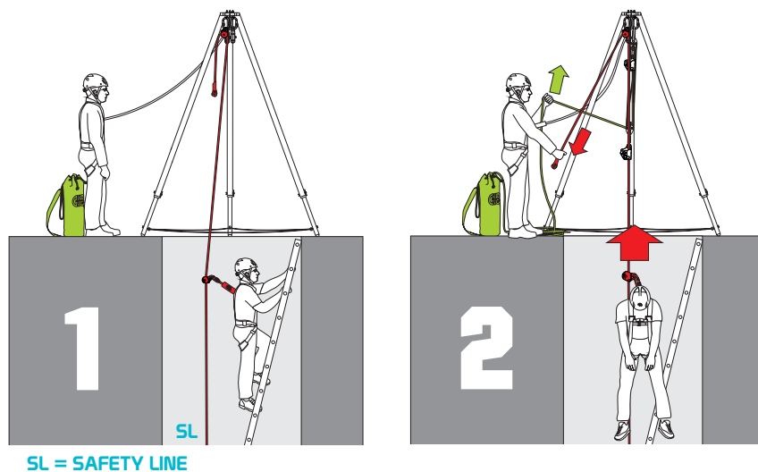
Fig. 5 – Esempio di corretto utilizzo - Accesso in ambiente confinato attrezzato con scala e della relativa evacuazione dell'operatore.
