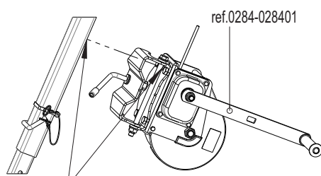
Den Sicherungsbolzen in einer Fixieröffnung des Stativbeins einbringen.
